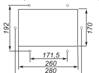
Plantilla para taladrar / Drill template
