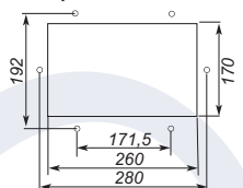
Plantilla para taladrar / Drill template
