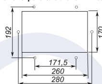
Plantilla para taladrar / Drill template
