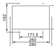
Plantilla para taladrar / Drill template
